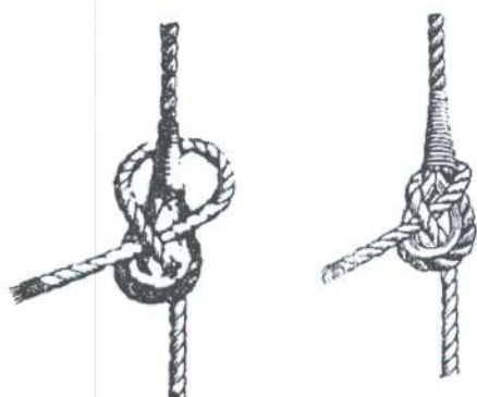
Шкотовый узел (на петле)
